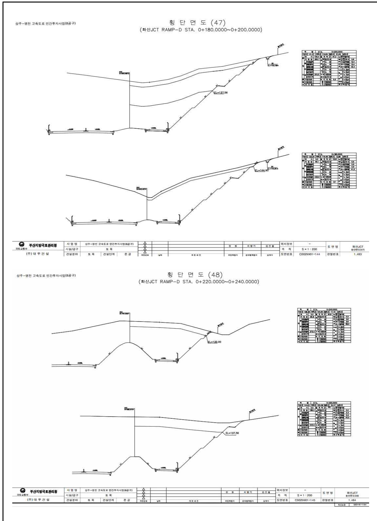
【그림 60.1.5】 표준횡단면도
